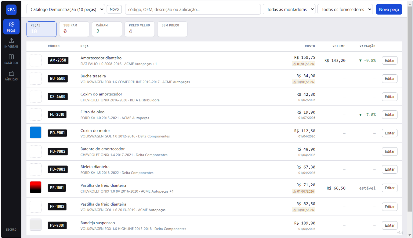
FIG. 03.1 A lista de peças é a tela. Na faixa escura à esquerda ficam as quatro seções; em cima, o catálogo em uso, a busca e os filtros; e a linha de contadores separa o que mudou de preço do resto.
